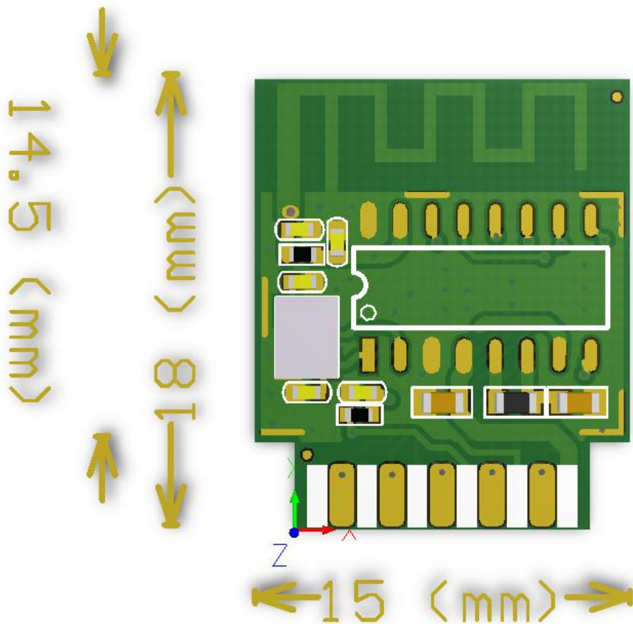
图 3 模组尺寸
