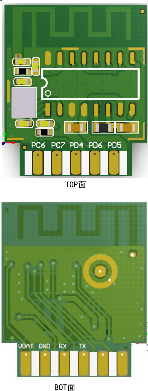
图 1 模块脚位分布图
