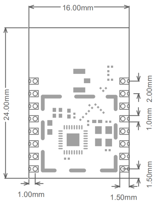
Figure 4. W-CB1S 机械尺寸
