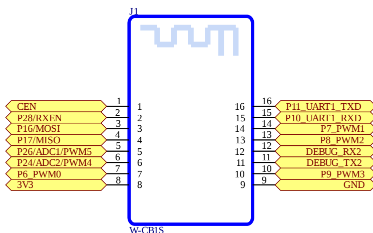
Figure 3. W-CB1S 管脚定义
