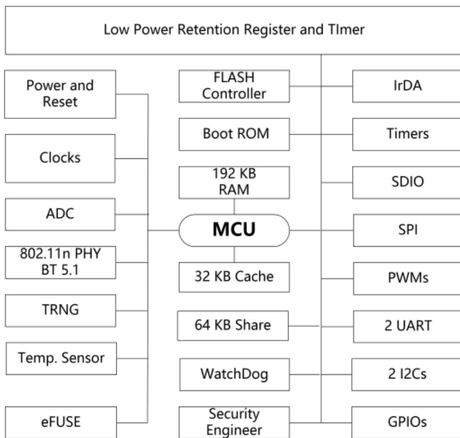
Figure 1. 系统框图
